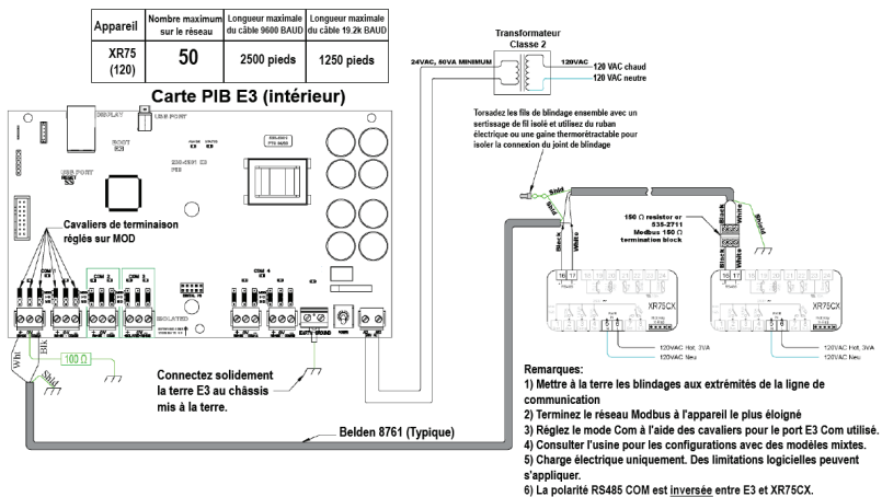
Câblage E3 et XR75
