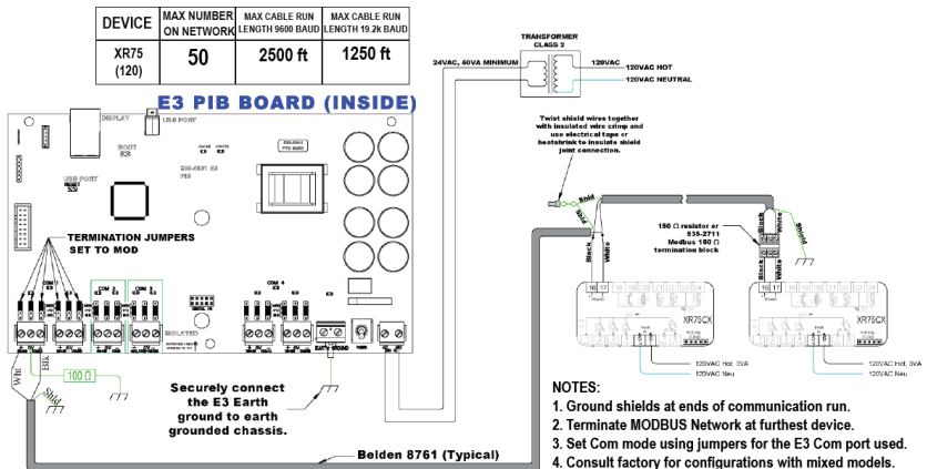
E3 and XR75 Wiring
